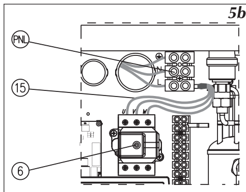
Рис.5б Подключение котла EKCO.M1 в трехфазную электрическую сеть (касается котлов 4 кВт, 6 кВт и 8 кВт).
