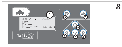
Рис.8 Панель управления ЕКСО.M1z/ ЕКСО.TM 1 - дисплей, 2-7 - клавиатура
