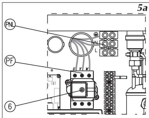
Рис.5а Подключение котла EKCO.M1 в однофазную электрическую сеть.
